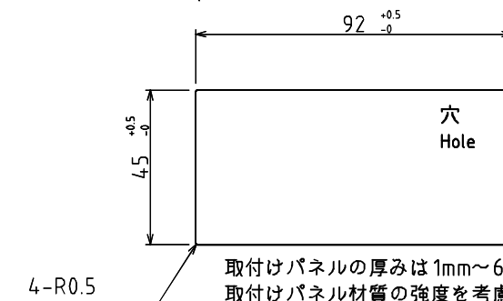
取付け穴寸法図
